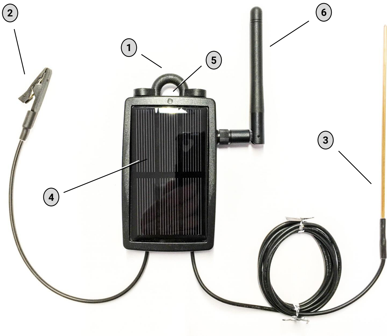
Abbildung 1: ZaunMonitor mit montierter Antenne
